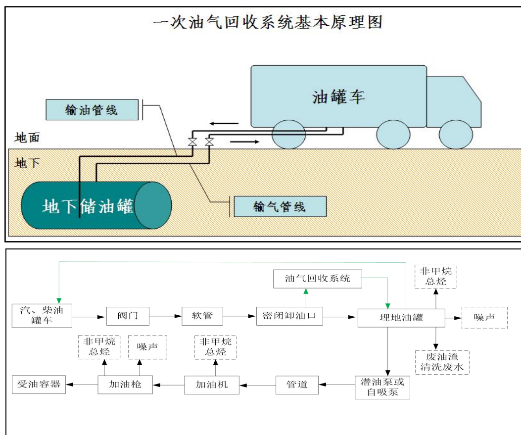
图2-3 项目工艺流程及产污环节图（一次油气回收装置）
